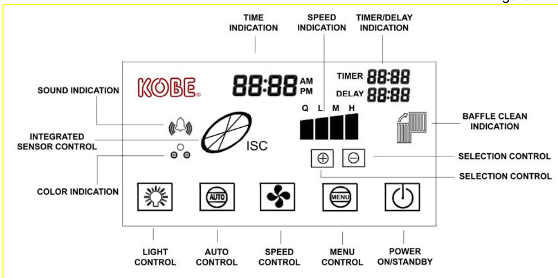
LCD DISPLAY
